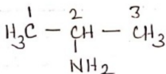
Propan-2-amine
