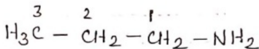
Propan-1-amine.
