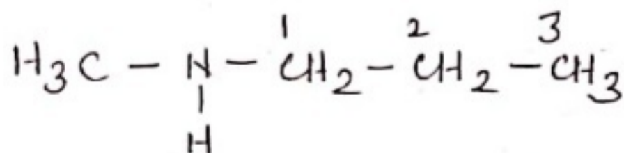
N-methylpropan-1-amine.
