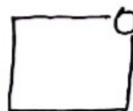
Oxetane
