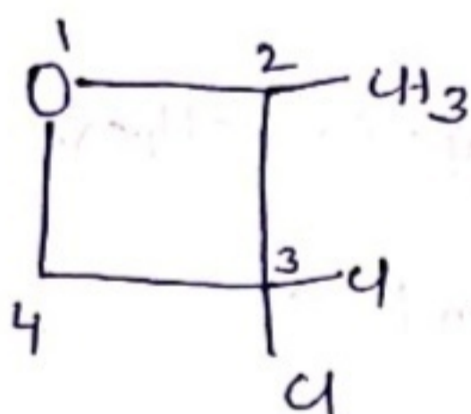
3,3-dichloro-2-methyloxetane
