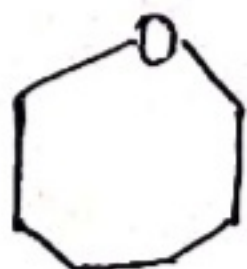
Oxepane
