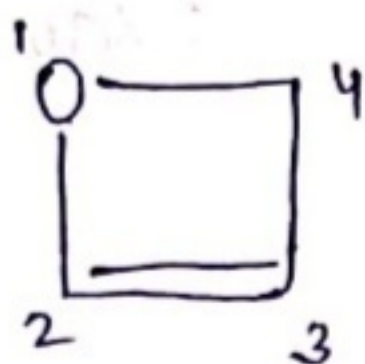
oxetene
