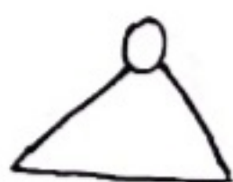
Oxirane
