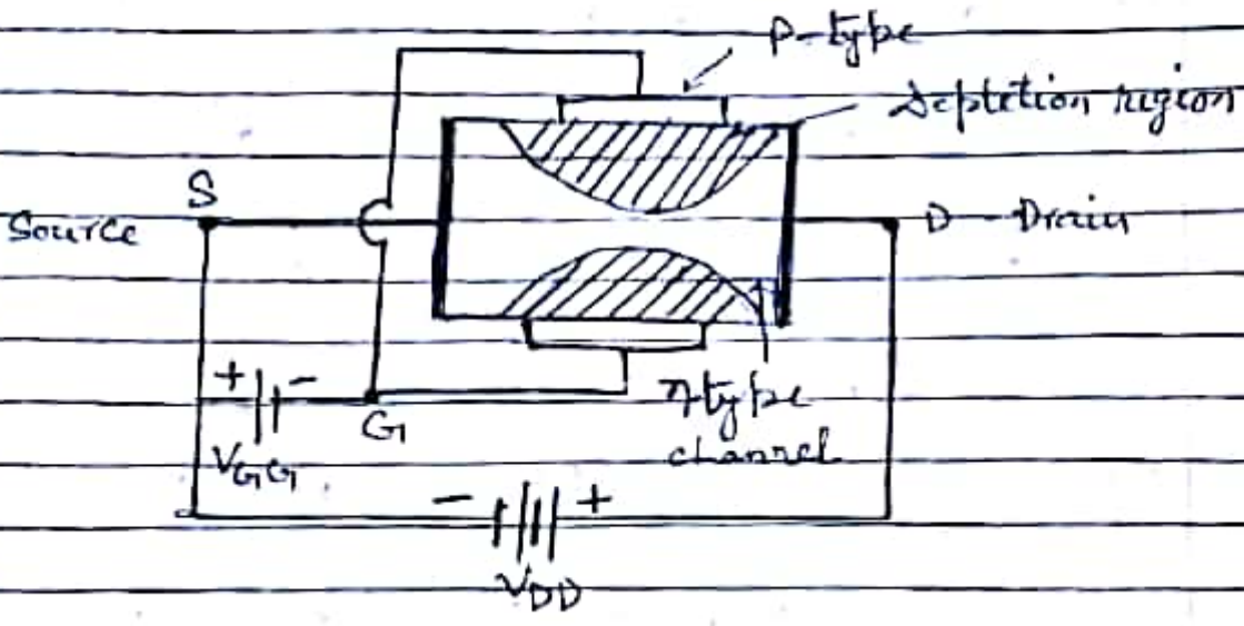
Fig. 1 A JFET
