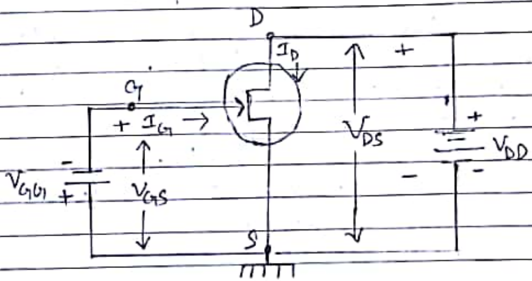
n-channel - FET
