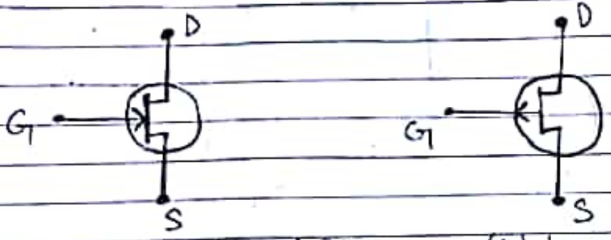
fig. 2 (a) n-channel FET. (b) p-channel FET
