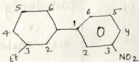
1-(3-ethylcyclohexyl)-3-nitrobenzene
